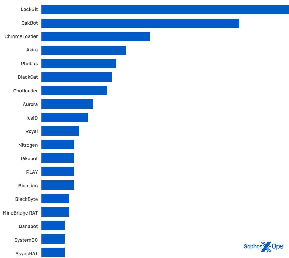
Figura 9: Malware observado con mayor frecuencia en incidentes gestionados por Sophos Managed Detection and Response en 2023, como se puede ver en el conjunto de datos de MDR. Fíjese en las diferencias entre este gráfico y el de la Figura 8: aparte de la prevalencia de LockBit en 2023, vemos que existe una amplia variedad de familias de ransomware que intentan infectar sistemas. Solo un subconjunto de ellas evolucionan hasta una fase que requiere la intervención de MDR. Tenga en cuenta que no son excluyentes; es decir, puede darse más de una detección en un único incidente.
